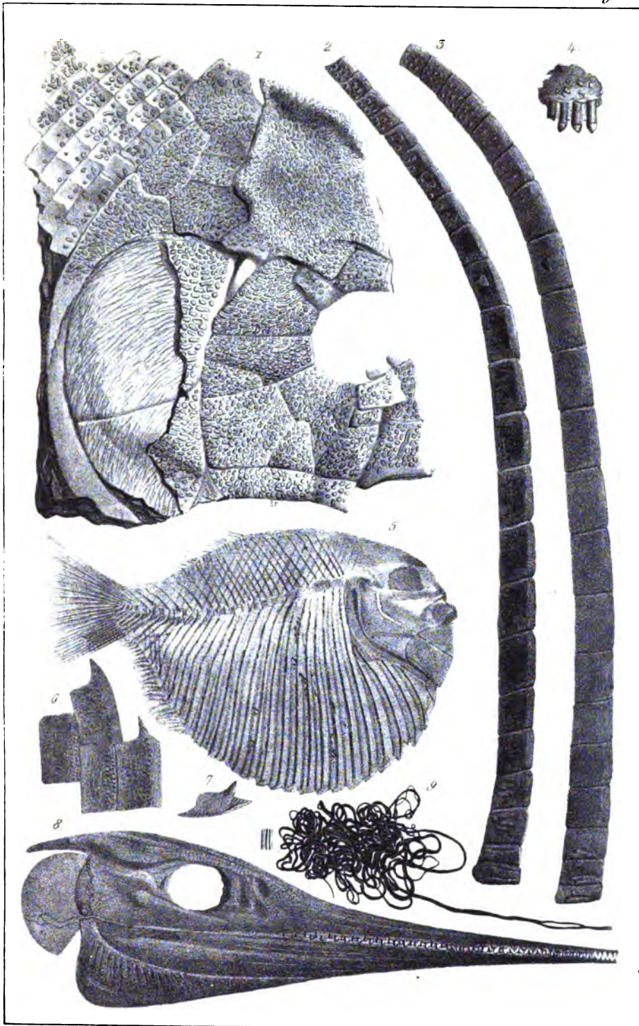
Quenstedt, Jura.
